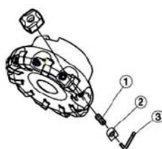
Keilspannpratze
