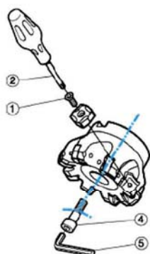
Schraubspann-System
